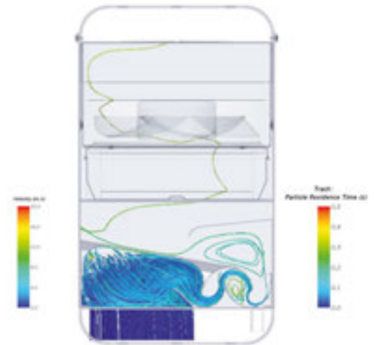
CFD-Bild 2: Verhalten der Partikel
